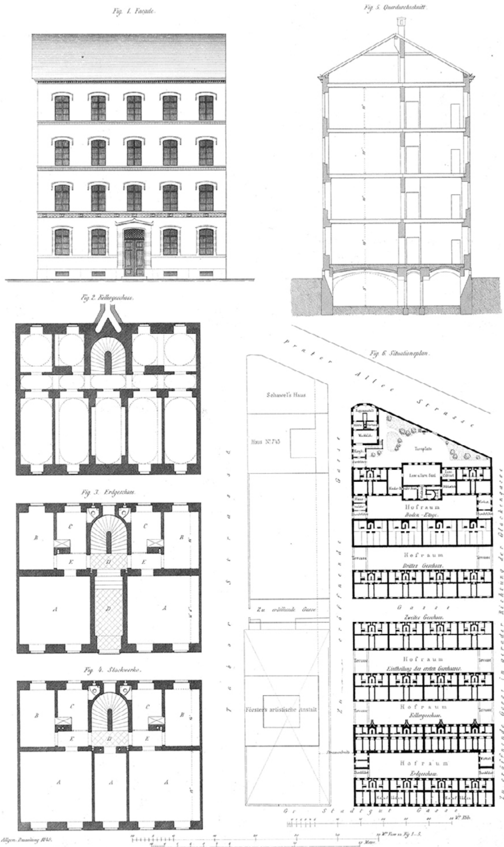
Kuva 3. Ludwig Försterin toimittamassaan lehdessä Allgemeine Bauzeitung esittelemä suunnitelma työväestön asuintaloksi Wieniin. Julkisivu-, leikkaus- ja pohjapiirustukset, Allgemeine Bauzeitung 1849, kuvataulu 263. Lähde: ANNO Historische österreichische Zeitungen und Zeitschriften.
